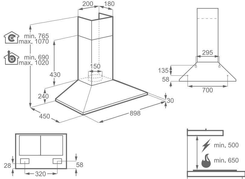
LFC319X Kürtős páraelszívó
