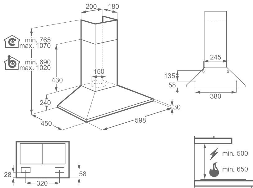
LFC316X Kürtős páraelszívó
